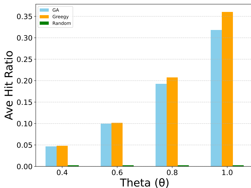
図 4.3: 平均キャッシュヒット率
