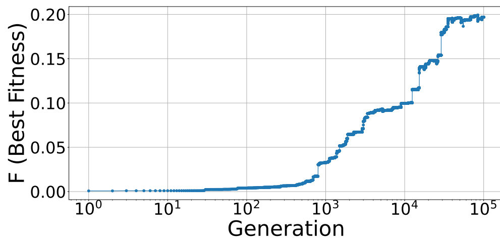
図 4.1: Result of GA(30)
