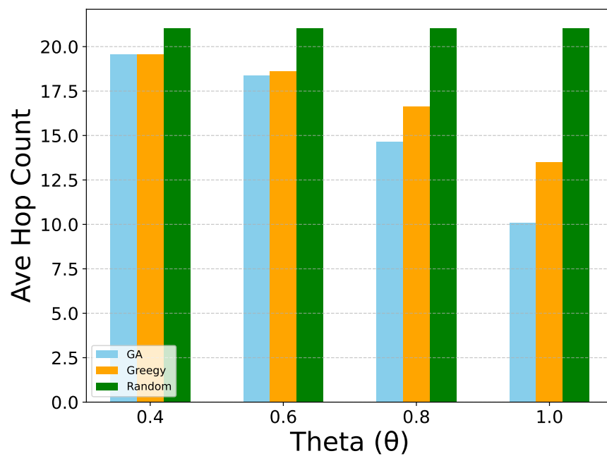
図 4.4: 平均ホップ数
