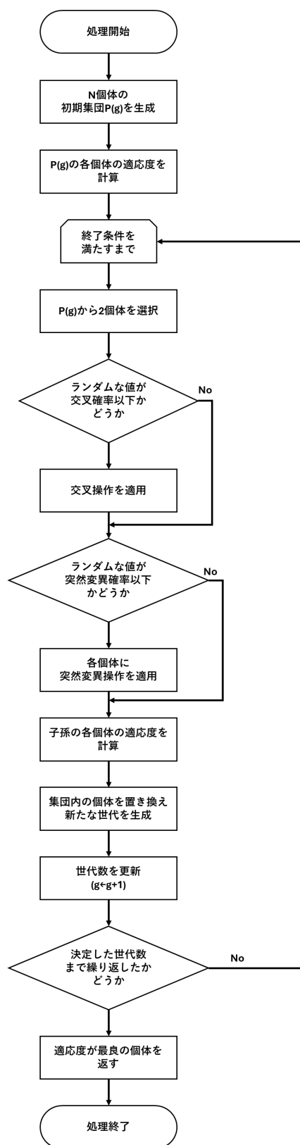
図 3.2: GA 処理チャート
