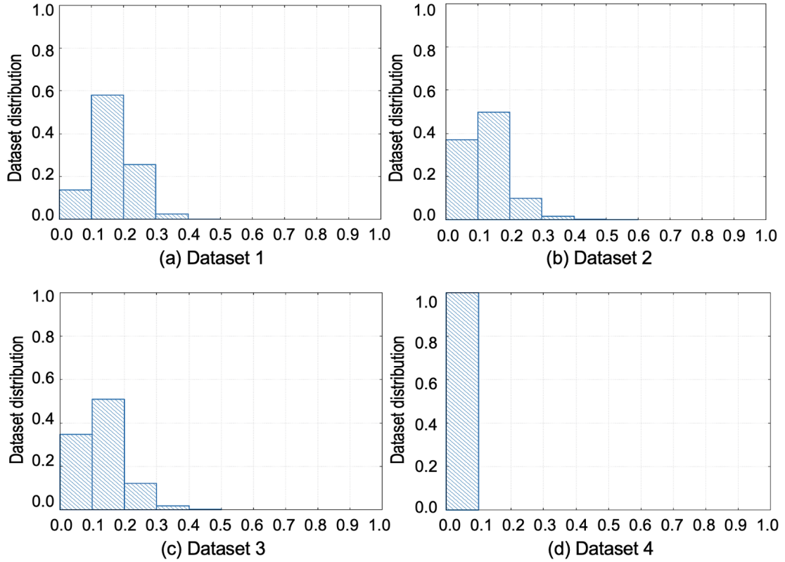
図 4.1: Dataset distribution
