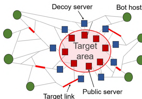
図 1 Crossfire Attack
